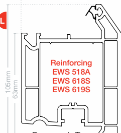
Door sash T EWS 7019
